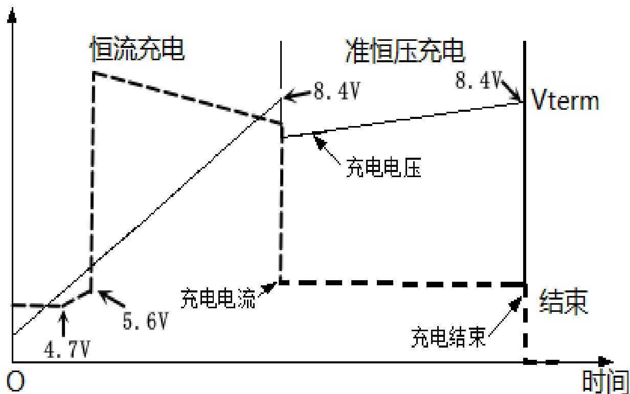
图4 充电过程
