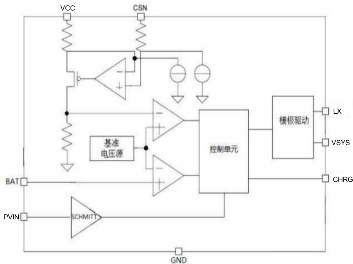
图 3 功能框图
