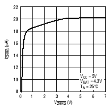
弱下拉状态下的 CHRG 引脚 I-V 曲线
