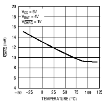
强下拉状态下的 CHRG 引脚电流与温度的关系曲线
